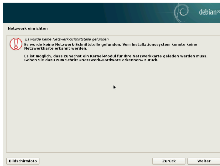
Abb. 5: Bestätigung Netzwerkkarte
