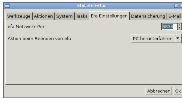
Abb. 29: Efa Einstellungen
