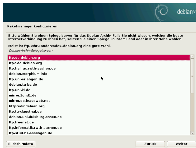
Abb. 15: Spiegelserver auswählen
